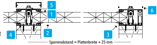
Verbindungsprofil
