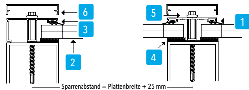
Verbindungsprofil
