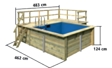
Abb. RECHTECKPOOL GRÖßE 3 inkl. Terrasse B, KDI, inkl. Bodenschutzvlies, Holzleiter und Edelstahlleiter
