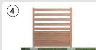
Füllprofile in die Pfostennuten einsetzen und ausrichten. Anschließend die Füllprofile in einem 45°-Winkel, mit Edelstahlsschrauben 4x50mm an den Pfosten fixieren.
