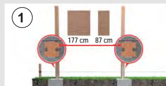
H-Anker bzw. EASY-FENCE ALU-Pfosten einbetonieren
