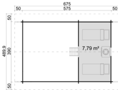
CAROLINE OBERGESCHOSS
