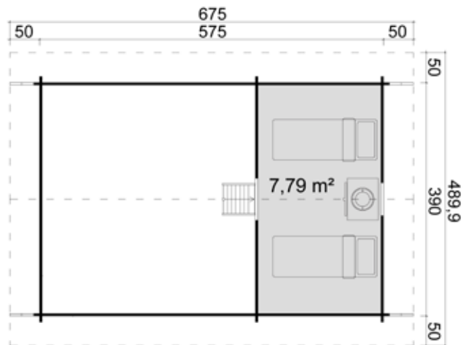
CAROLINE 2.3 OBERGESCHOSS
