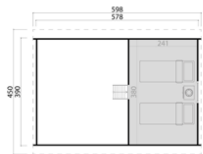
MURANO 3 OBERGESCHOSS
