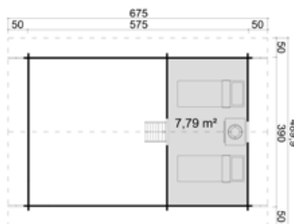
CAROLINE 2.2 OBERGESCHOSS
