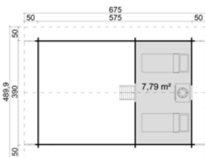
CAROLINE 2.1 OBERGESCHOSS
