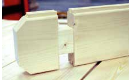
Winddichte Chaletschnitt-Eckverbindung
